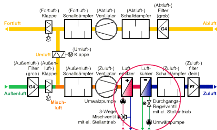
Zu- und Abluftschema einer Teilklimaanlage
