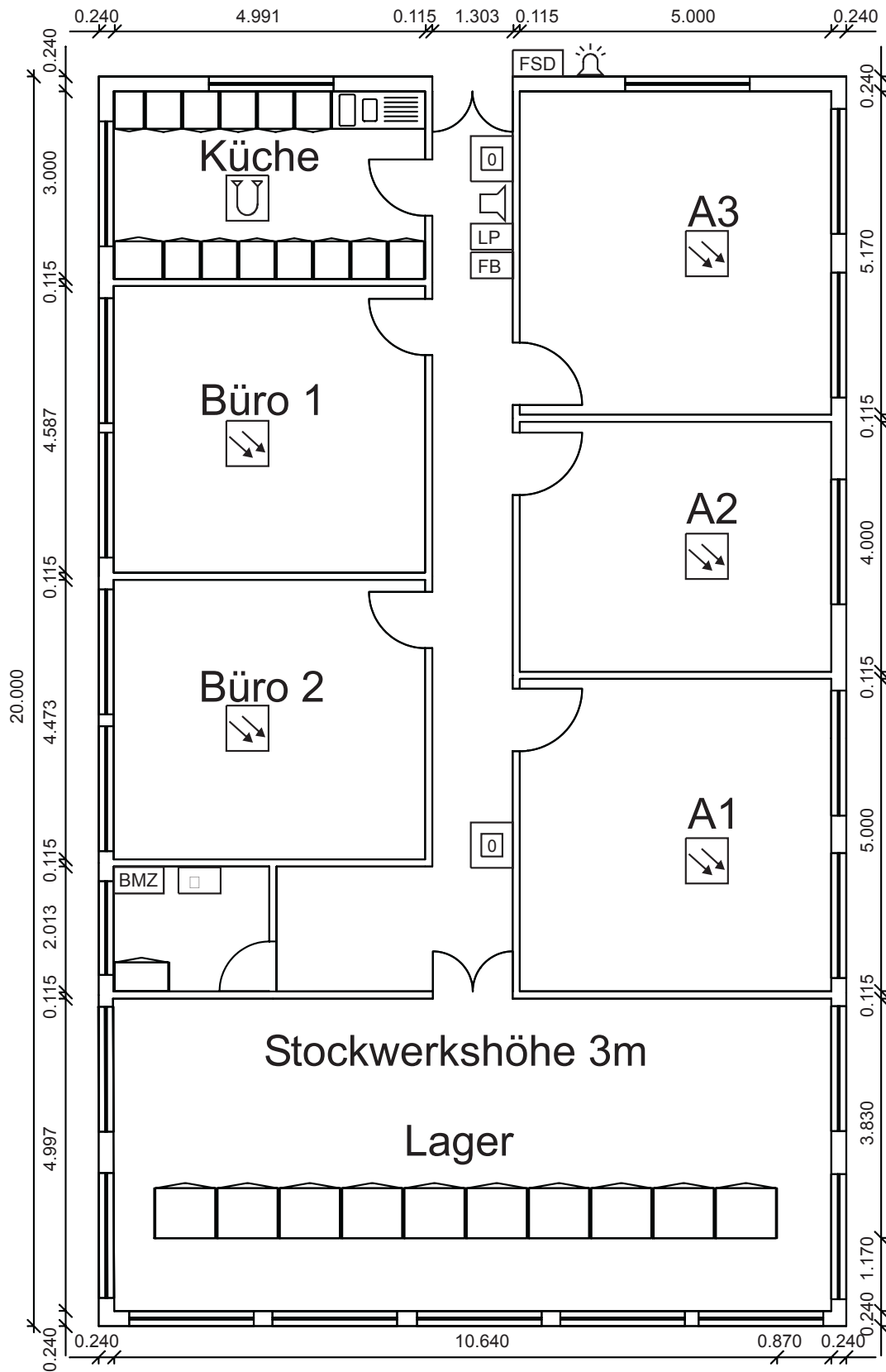
Bild: Grundriss (Raumhöhe 3m, Flachdach)
