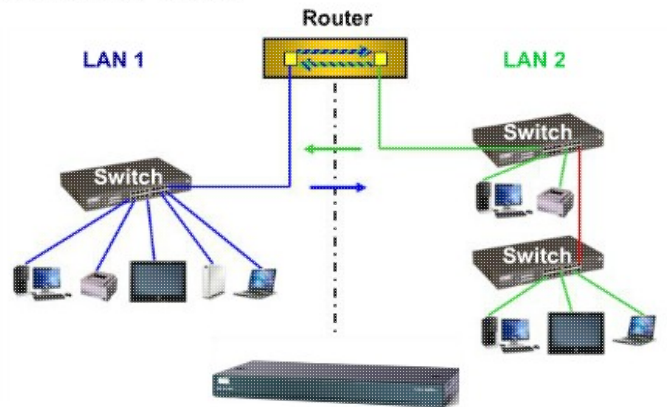
Netzverbinder - Router
