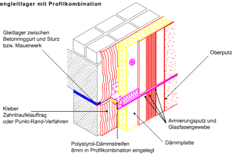
Deckengleitlager mit Profilkombination
