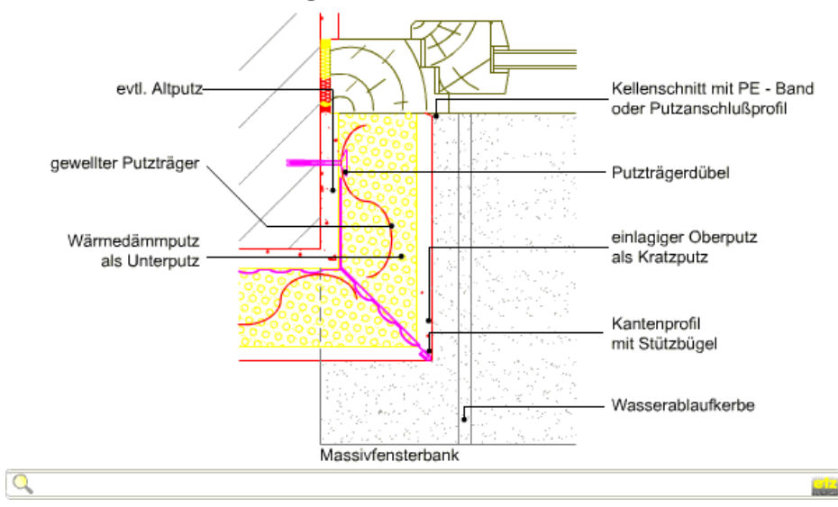
WDVS Fensteranschluss mit Fugendichtband
