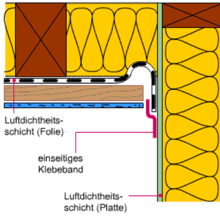
b) Wandanschluss
