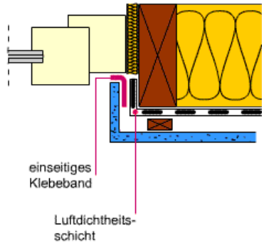
a) Fensteranschluss
