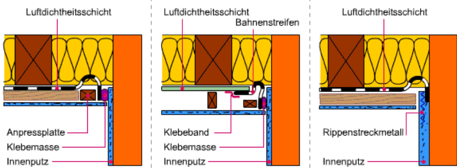
Anschluss mit komprimiertem Dichtband bzw. geeigneter Klebmasse und verschraubter Anpressplatte
