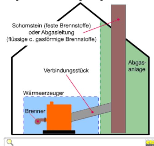
Begriffe einer Feuerungsanlage
