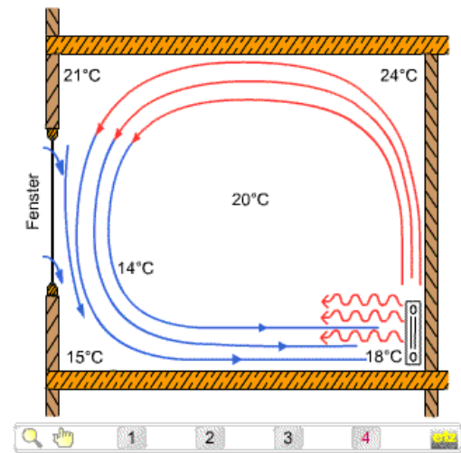
Heizkörperanordnung an einer Innenwand bei unausgeglichene Raumlufthtemperaturen
