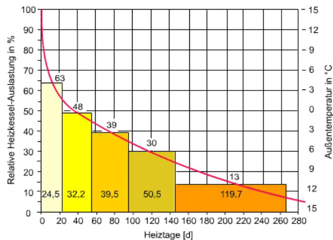
Jahresdauerkennlinie
