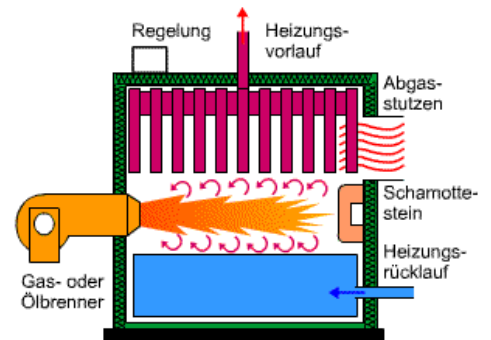
Gusskessel aus aneinandergereihten Hohlkörpern
